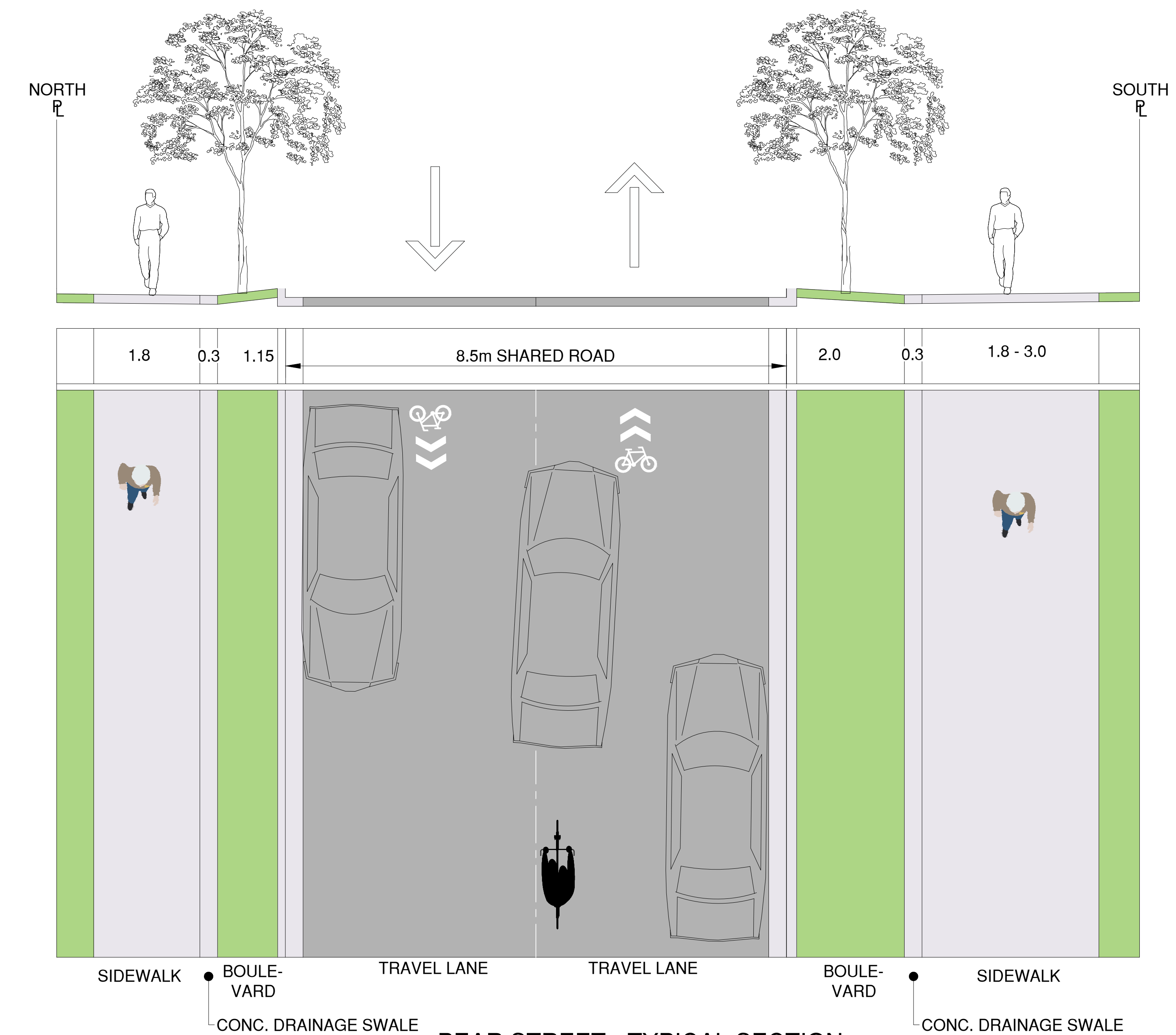
PEAR STREET - TYPICAL SECTION SCALE: N.T.S.
